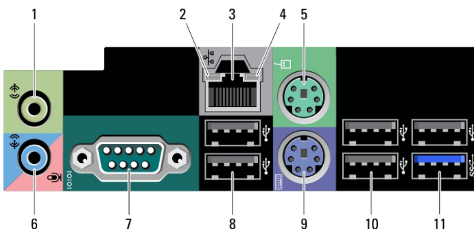
Figura2. Vista do painel posterior
